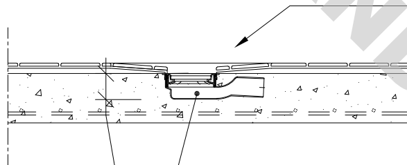
SEKTIONSSNITT
